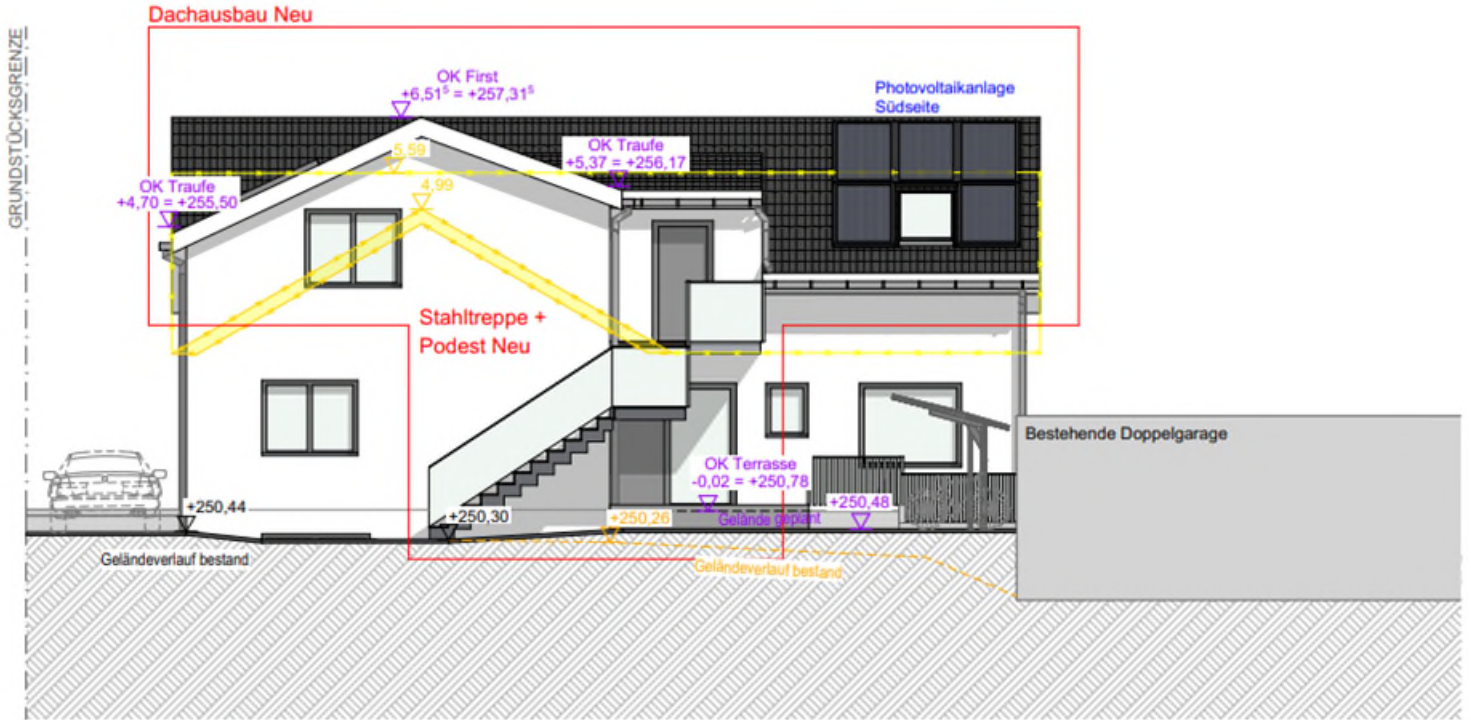
ansicht süd
