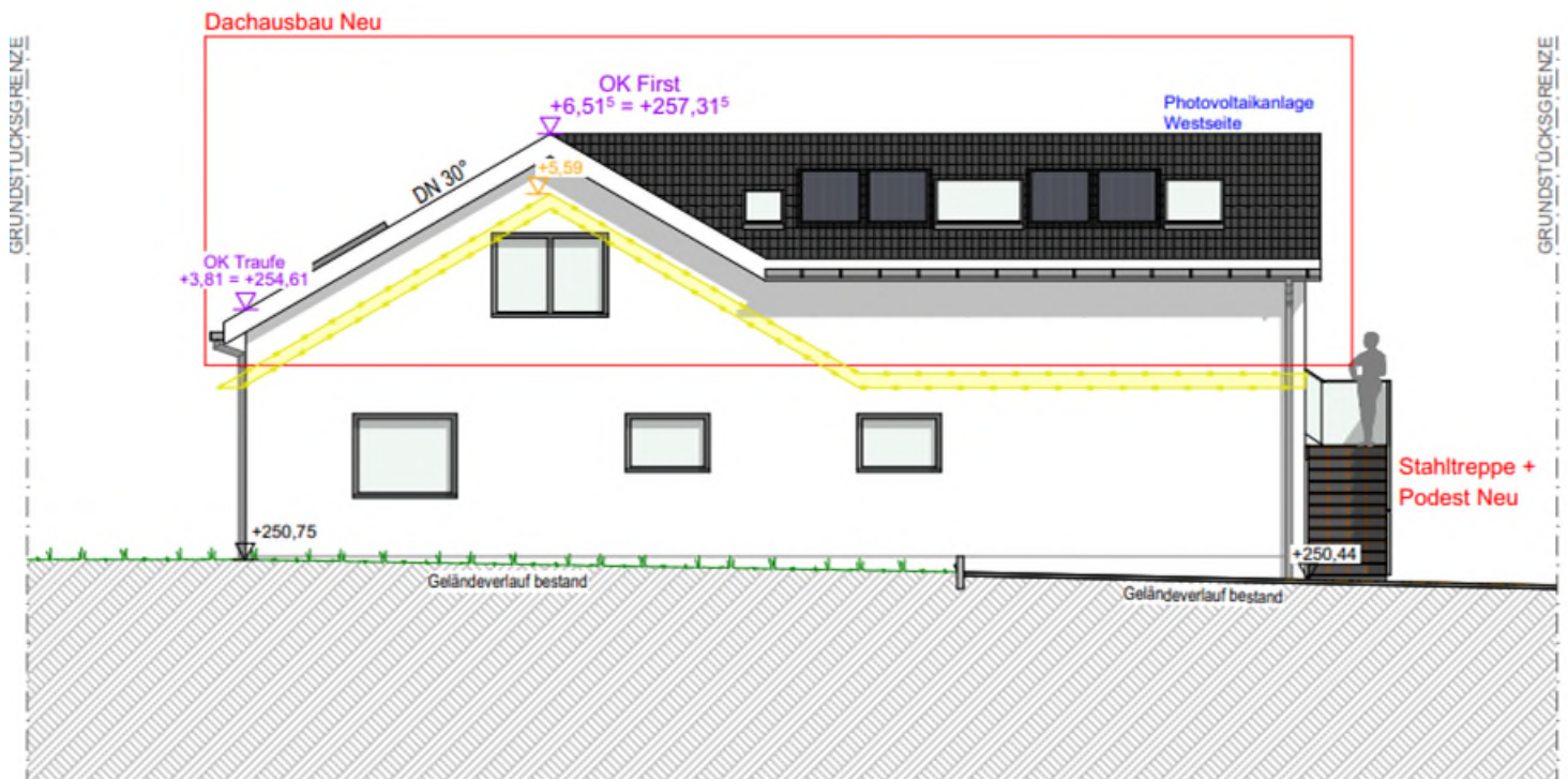
ansicht west
