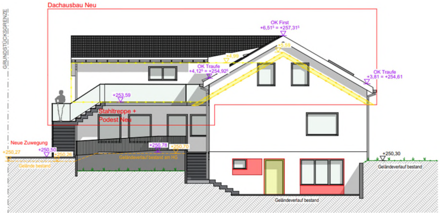
ansicht ost
