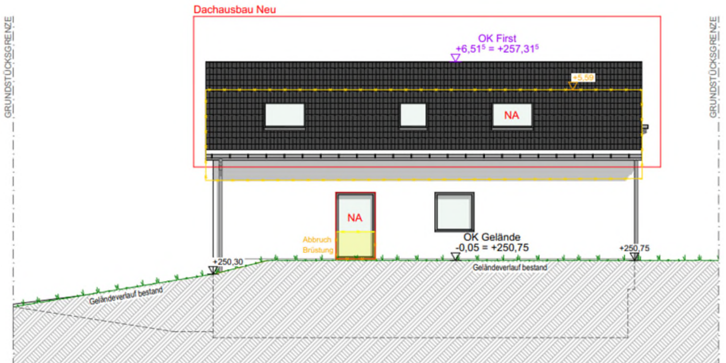
ansicht nord
