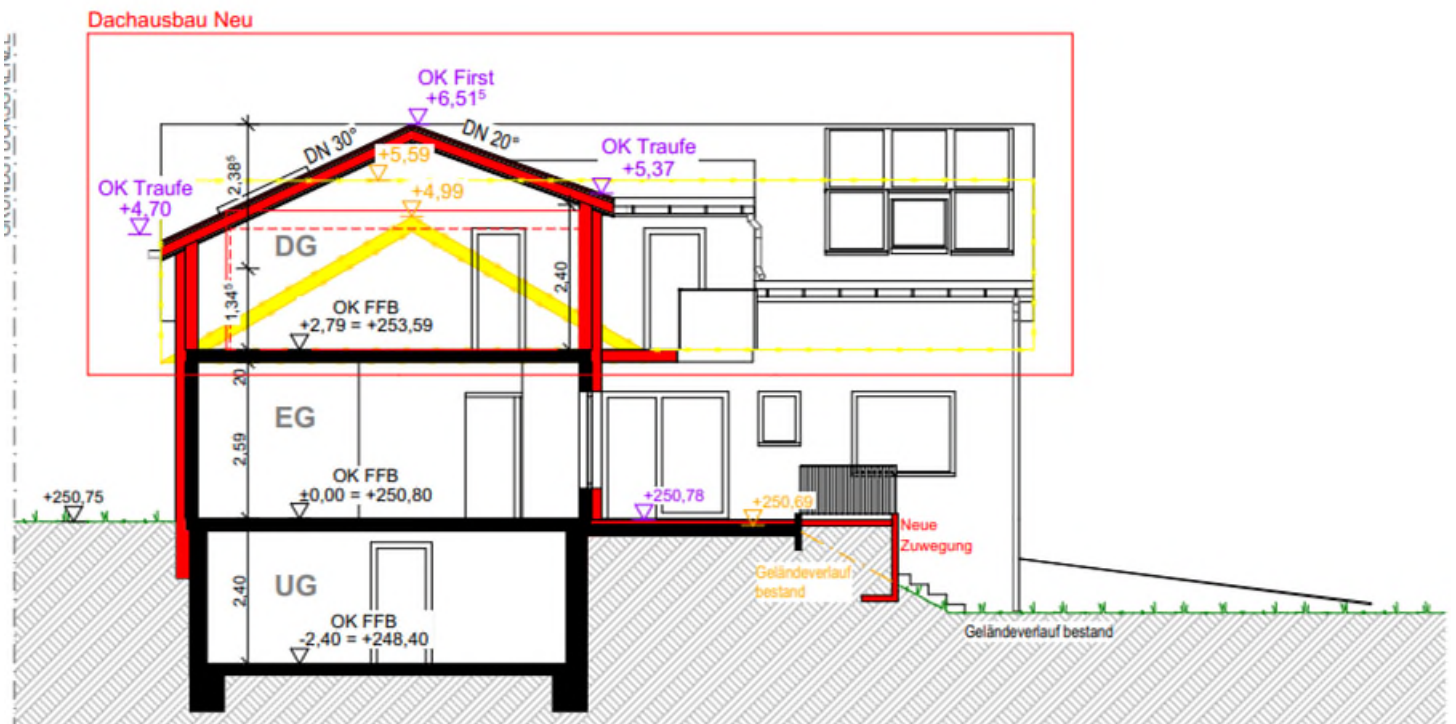
schnitt b-b
